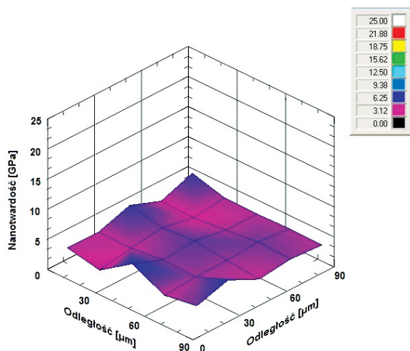
Rys. 8. Rozkład 3D nanotwardości próbki referencyjnej MR
