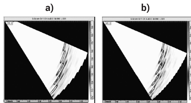
Rys. 4. Skan sektorowy ze wskazaniami od jednakowych otworów poprzecznych usytuowanych w różnych miejscach próbki uzyskany a) przed oraz b) po wykonaniu kalibracji ACG i TCG Fig. 4. Sectorial scans with indications from identical side drilled holes situated at different depths of reference block registered a) before and b) after ACG and TCG calibrations
