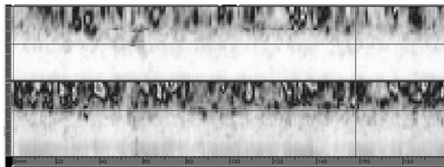
Rys. 8. Przykład zobrazowań typu C z dwóch głowic PA umieszczonych po przeciwnych stronach spoiny
