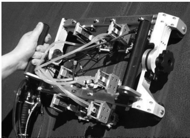
Rys. 7. Ręczny skaner HSMT-Flex firmy Olympus do badań złączy spawanych techniką PA oraz TOFD
