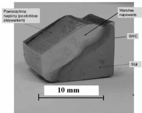
Rys. 5. Przekrój warstwy napawanej Fig. 5. Cross-section of the padding weld
