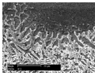
Rys. 7. SEM; mikrostruktura napoiny w miejscu nakładania się ściegów
