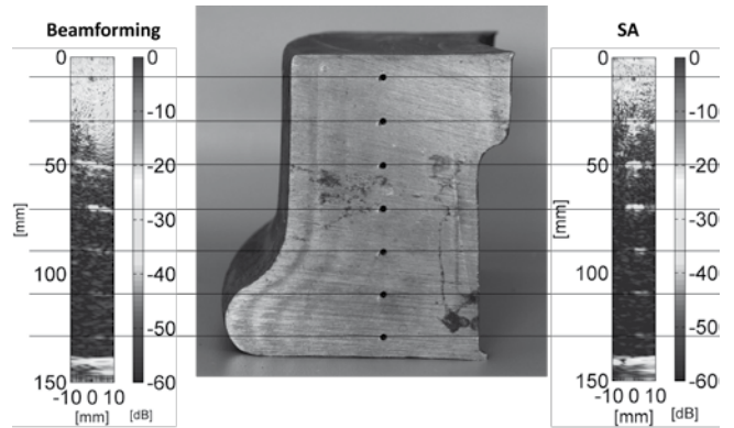
Rys. 2. Obraz wad w monobloku uzyskany metodą beamformingu oraz syntetycznej apertury
